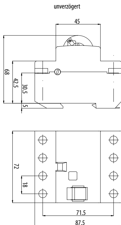
K-kurzzeitverzögert, S-selektiv
