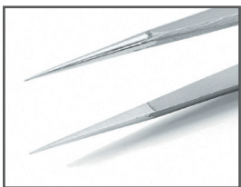
00 ion
