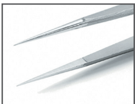
SS ion
