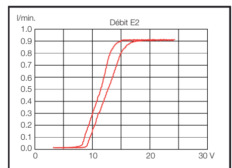
Courbe Typique d'Hystérésis pour les débits de 0 à 90 l/min
