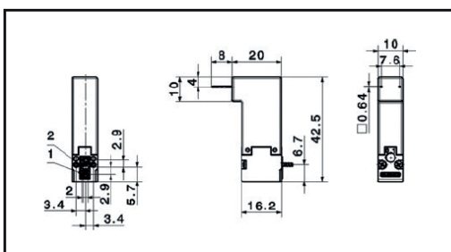
Vanne proportionnelle Kuhnke de la série 63P
